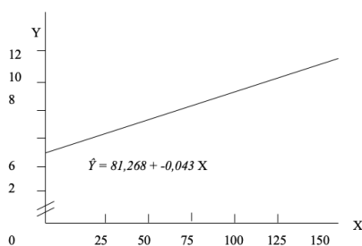
Gambar 5. Grafik Garis Regresi \hat{Y} = 81,268 + -0,043 X
